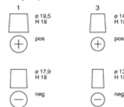
Priključni polovi
