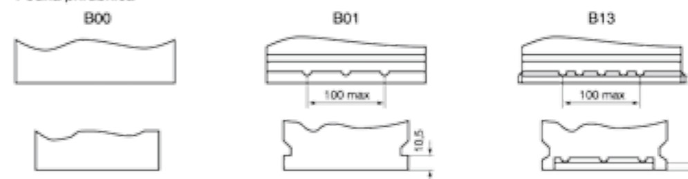
Podna prirubnica
