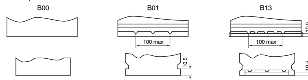
Podna prirubnica
