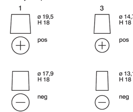
Priključni polovi
